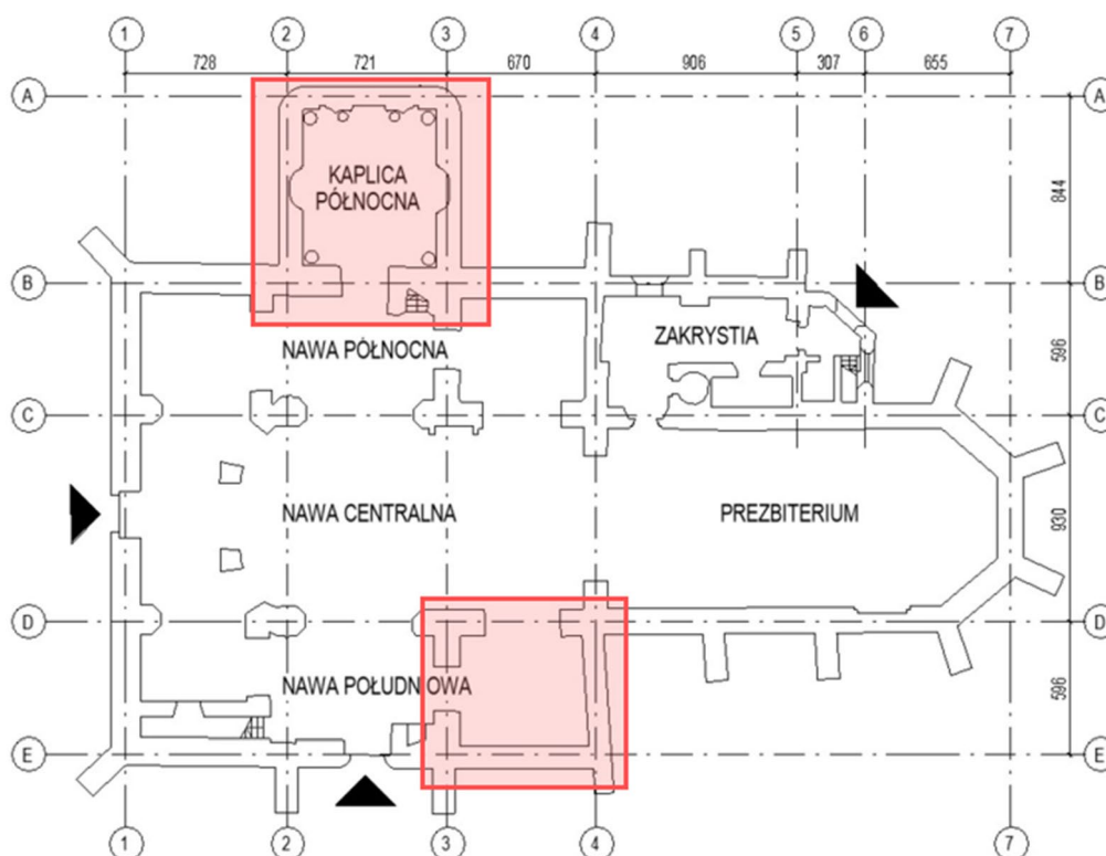
Rzut kościoła z oznaczeniem obszarów największych uszkodzeń
